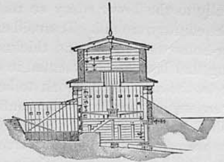
FIG. 3. SECTION ON A. B. (FIG. 1.)
