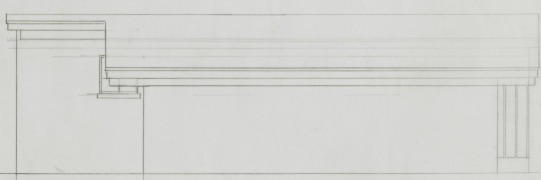
LEFT SIDE ELEV.
