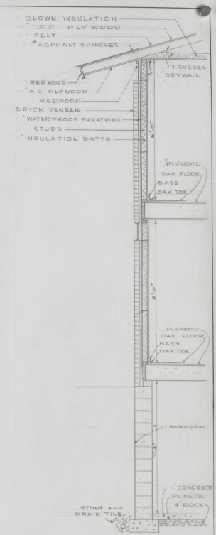
SECTION SCALE: 1/2" = 1'-0"
