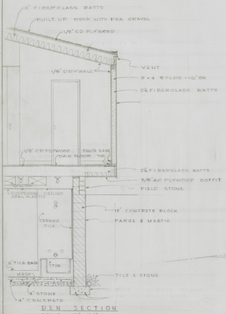
DEN SECTION SCALE: 1/8" = 1'-0"
