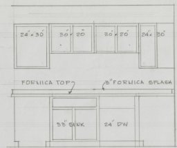
ELEV. B
